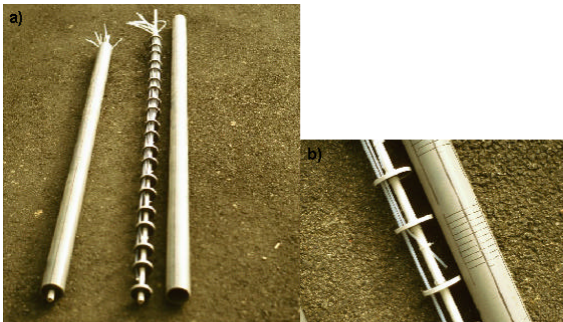
Figure 2.16 : Piézomètre compartimenté désossé a) vue d'ensemble b) détail d'un compartiment.
