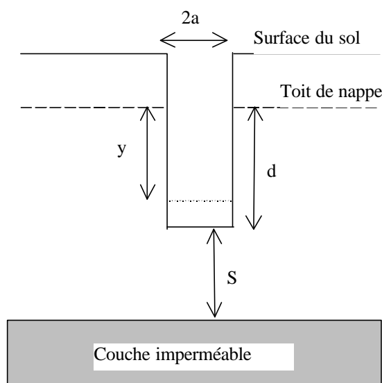
Figure 2.14 : Paramètres intervenant dans le calcul de la conductivité hydraulique à saturation ( K_{sat} ) par la méthode du trou de tarière.
