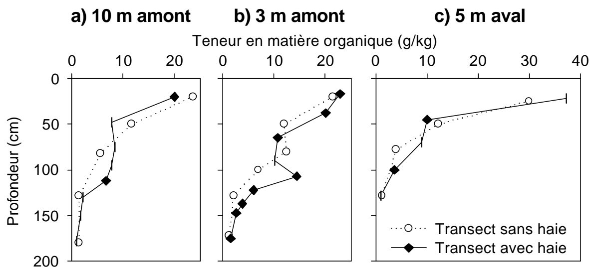
Figure 4.29 : Teneurs en matière organique a) à 10 m et b) à 3 m en amont et c) à 5 m en aval des deux transects
