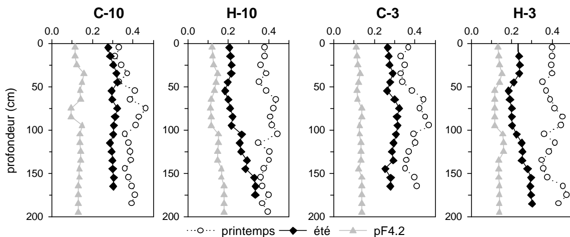
Figure 3.10 : Humidité volumique à 10 m (-10) à 3 m (-3) en amont des transects sans haie (C) et avec haie (H), début mai 99, fin août 99, et au point de flétrissement (pF 4.2).
