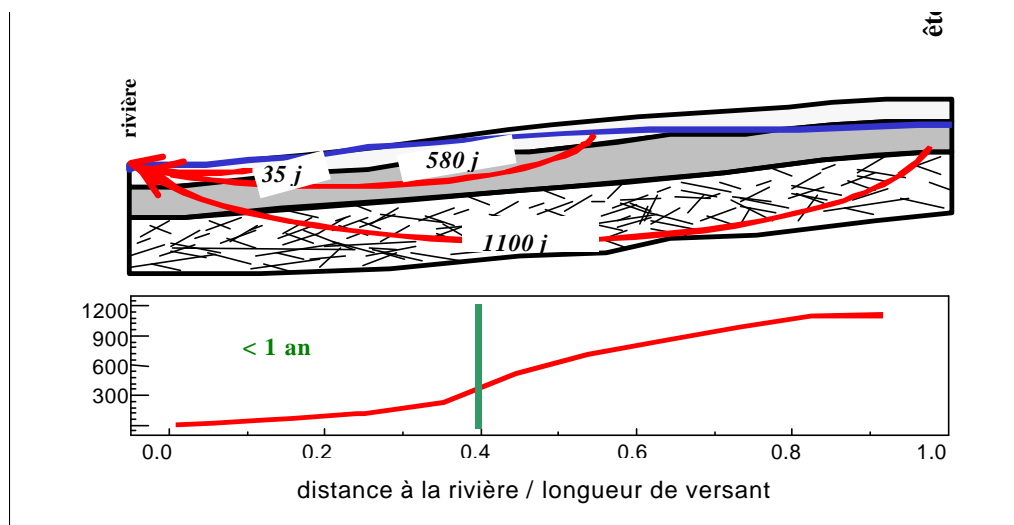
Figure 1.4 : Temps de résidence moyen de l'eau dans le sol le long d'un versant sur schiste. Bassin versant de Naizin (56). Molénat, 1999.
