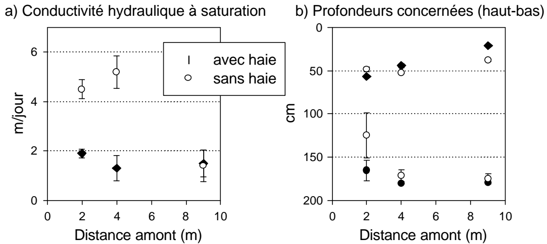
Figure 3.15 : a) Conductivités hydrauliques à saturation et b) profondeurs concernées (toit de nappe - base du sondage), mesurées en janvier 99 sur 5 répétitions.
