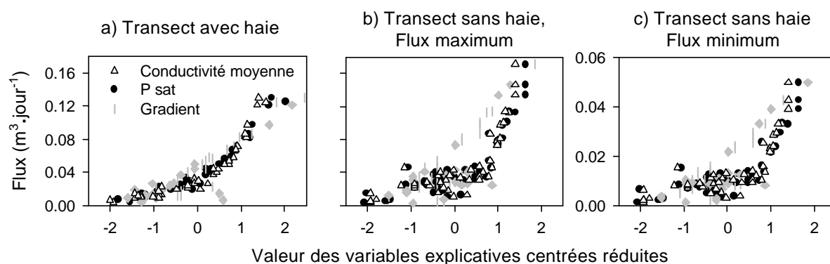
Figure 3.23 : Relation entre le flux et les différentes variables centrées réduites.
