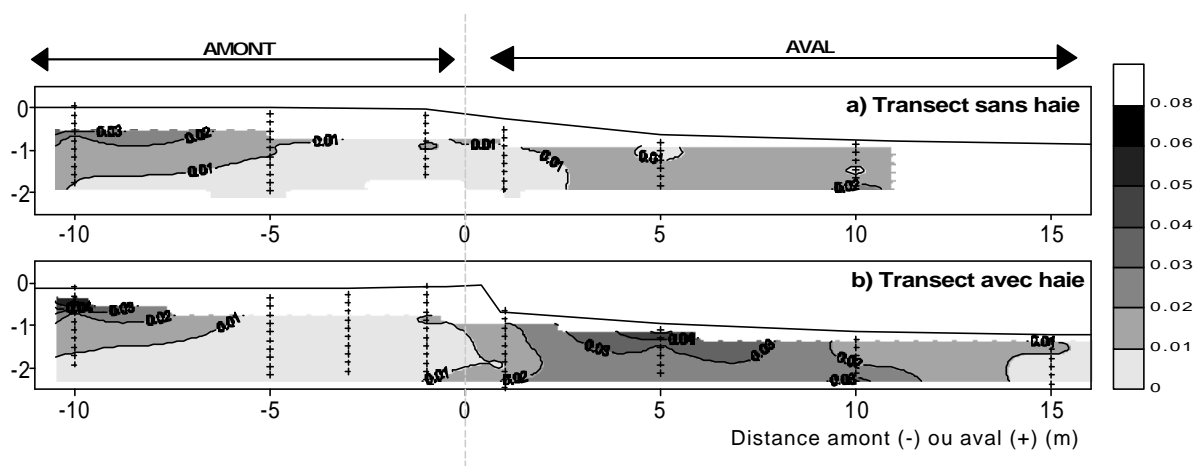
Figure 4.16 : Carte des isovaleurs de concentration en potassium dans la nappe le 11/02/99 a) sur le transect sans haie et b) sur le transect avec haie.
