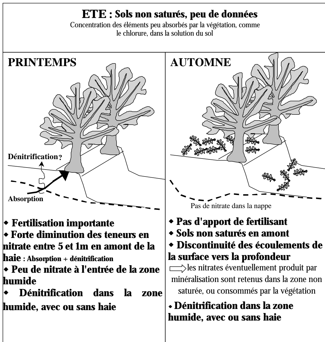
Figure 4.30 : Résumé de l'influence de la haie sur la dynamique et le transfert du nitrate dans la nappe.
