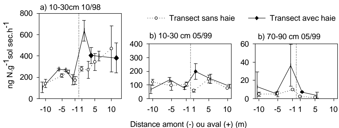
Figure 4.25 : Vitesses potentielles de dénitrification a) à 10-30 cm de profondeur en octobre 98 b) à 10-30 cm de profondeur en mai 99 et c) à 70-90 cm de profondeur en mai 99. Moyenne et écart type sur 5 répétitions.
