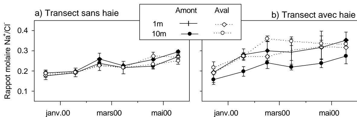
Figure 4.24 : Evolution du rapport molaire \text{Na}^+/\text{Cl}^- a) sur le transect sans haie et b) sur le transect avec haie de décembre 00 à mai 00. Moyenne et écart-type sur l'ensemble de la profondeur saturée.
