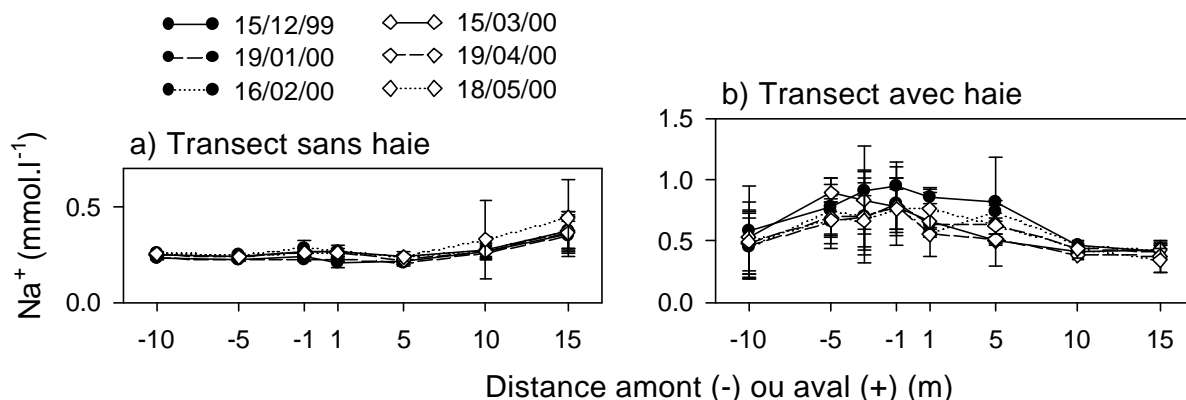
Figure 4.20 : Evolution des concentrations en sodium le long a) du transect sans haie et b) du transect avec haie de décembre 99 à mai 00. Moyenne et écart type dans chaque piézomètre compartimenté.
