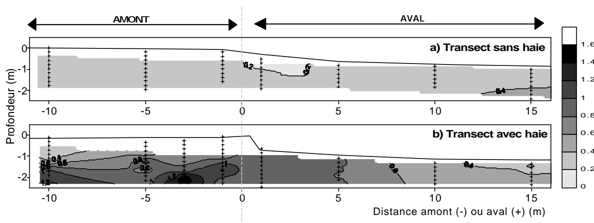
Figure 4.19 : Carte des isovaleurs de concentration en sodium dans la nappe le 15/12/99 a) sur le transect sans haie et b) sur le transect avec haie.
