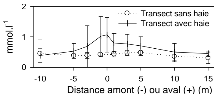
Figure 4.18 : Concentrations en sulfate le long des deux transects. Moyenne et écart type de mars 98 à avril 99.
