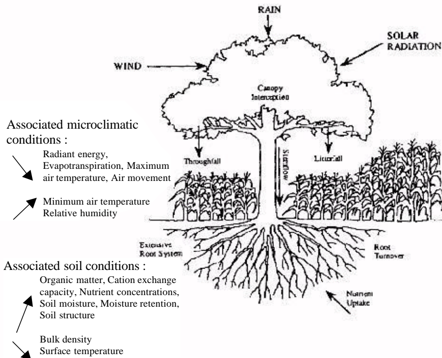
Figure 1.6 : Synthèse des facteurs influençant le fonctionnement du sol sous la canopée d'arbres isolés dans les systèmes agroforestiers mexicains (Farell, 1990, in Rhoades, 1997).
