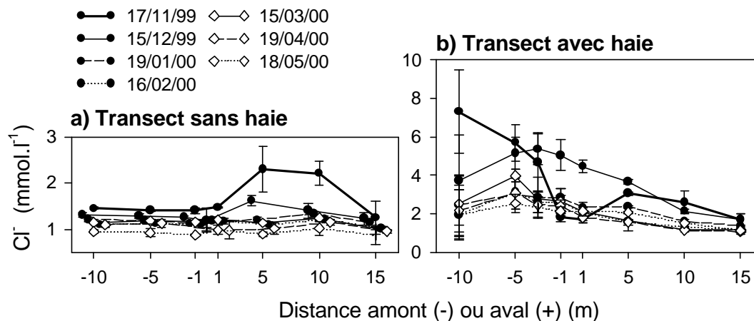
Figure 4.13 : Evolution des concentrations en chlorure le long a) du transect sans haie et b) du transect avec haie de novembre 99 à mai 00. Moyenne et écart type dans chaque piézomètre compartimenté.
