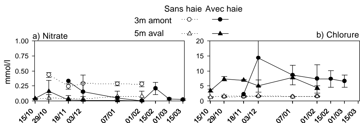
Figure 4.3 : Variabilité spatiale de la teneur a) en nitrate et b) en chlorure dans la nappe en amont et en aval des deux transects à différentes dates entre octobre 98 et mars 99. Moyenne et écart type sur trois piézomètres voisins.
